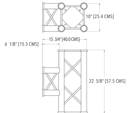
▶ TRL 009 TRUSS TEE
